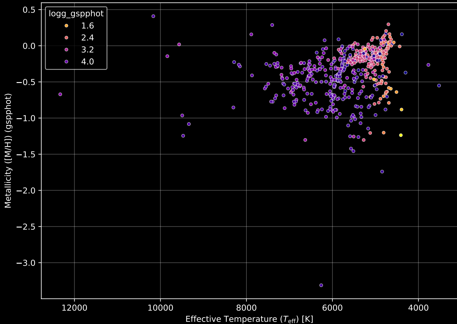
GALAH DR4 Field: [6778] Stellar Population Parameters (n= 503)
