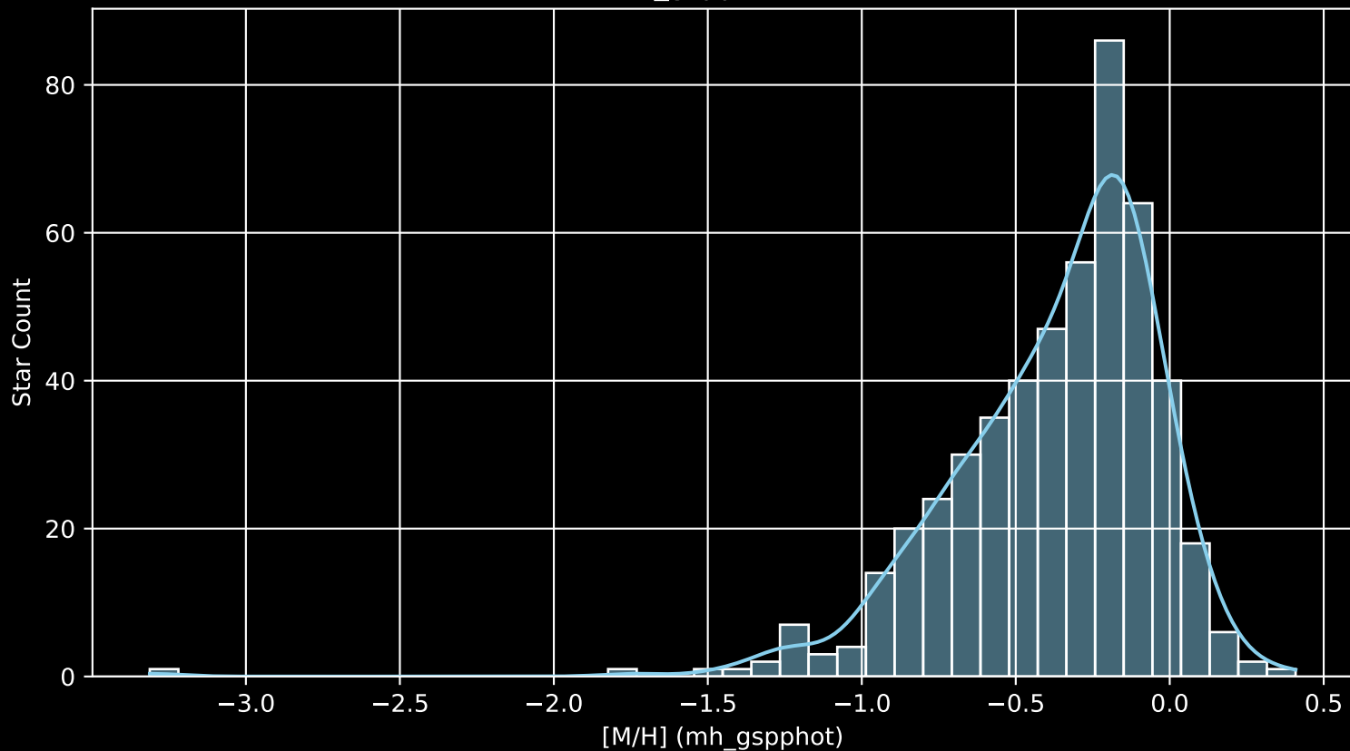
GALAH DR4 Field: [6778] [M/H] (mh_gspphot) (n= 503)
