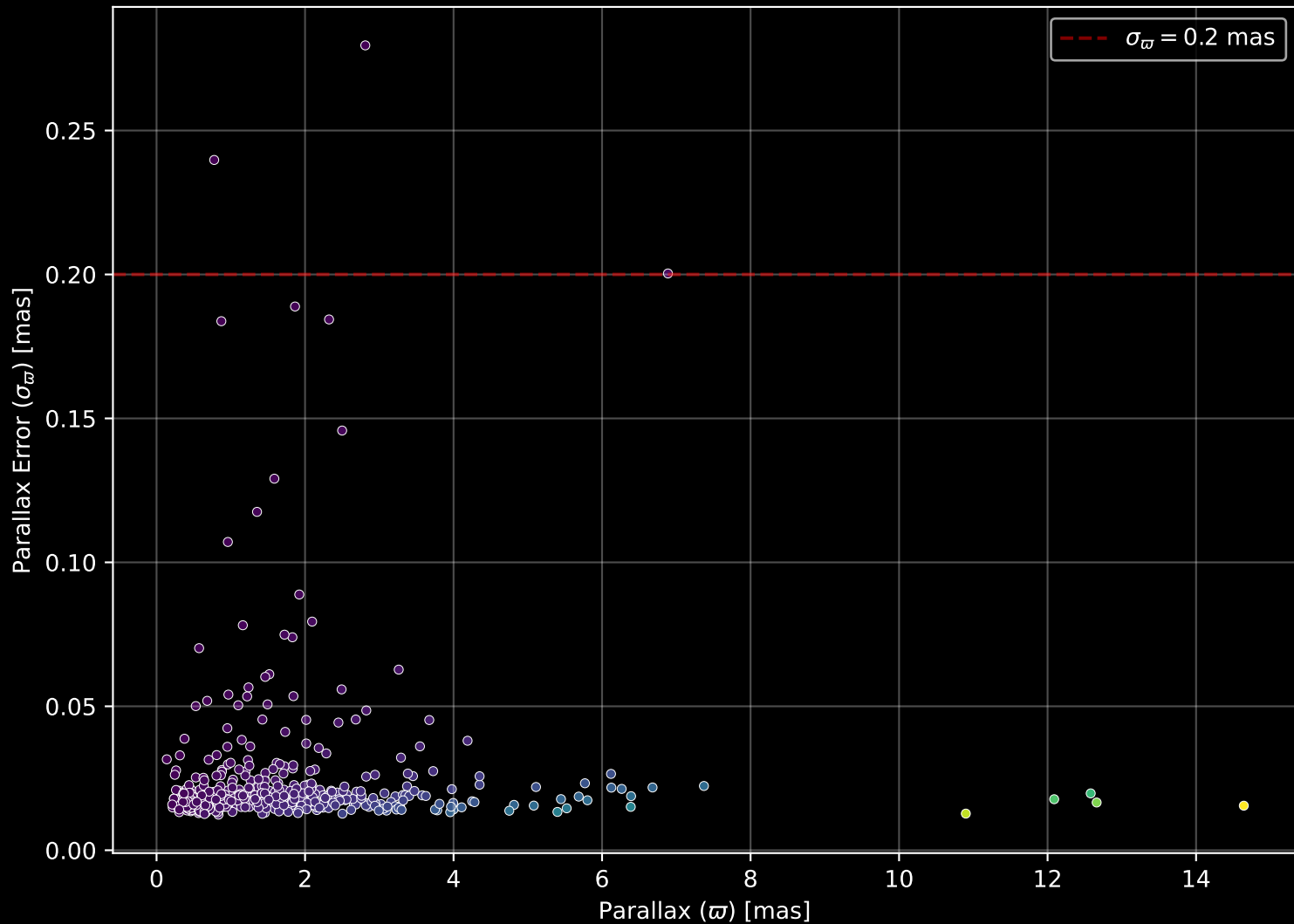
GALAH DR4 Field: [6778] Parallax Quality (n= 503)
